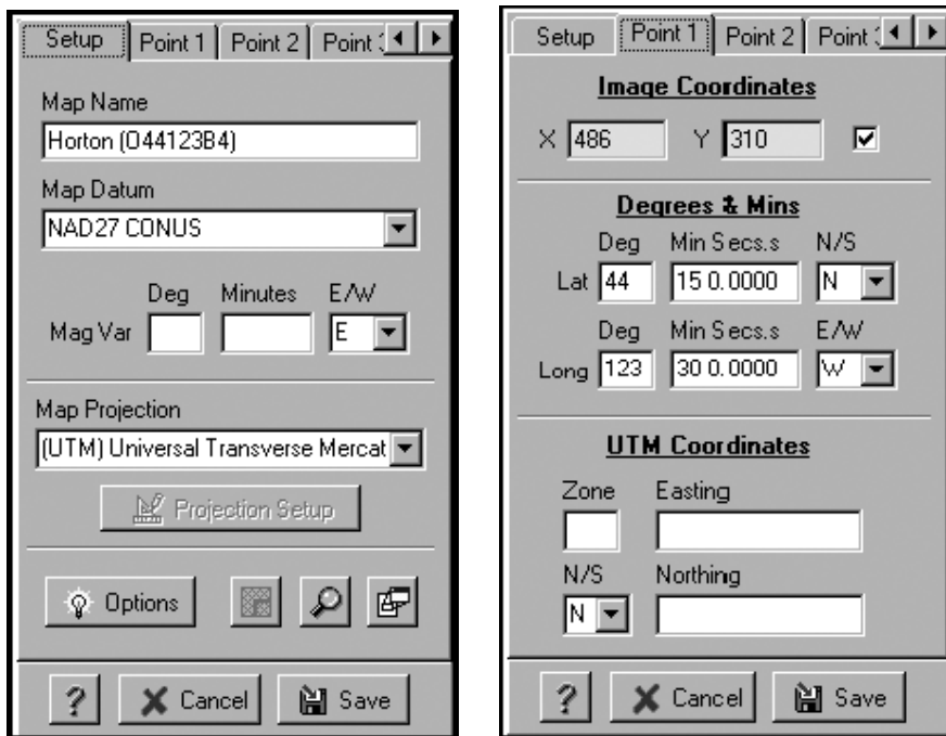
Рис. 3.19. Окна калибровки карты
