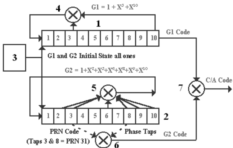
Рис. 2.6. Схема формирования С/А кода
