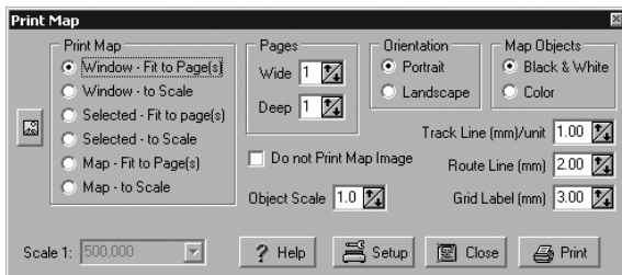
Рис. 3.21. Окно настройки печати карты
