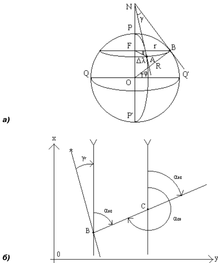
Рис. 1.8. К определению сближения меридианов (а) и дирекционного (б) угла
