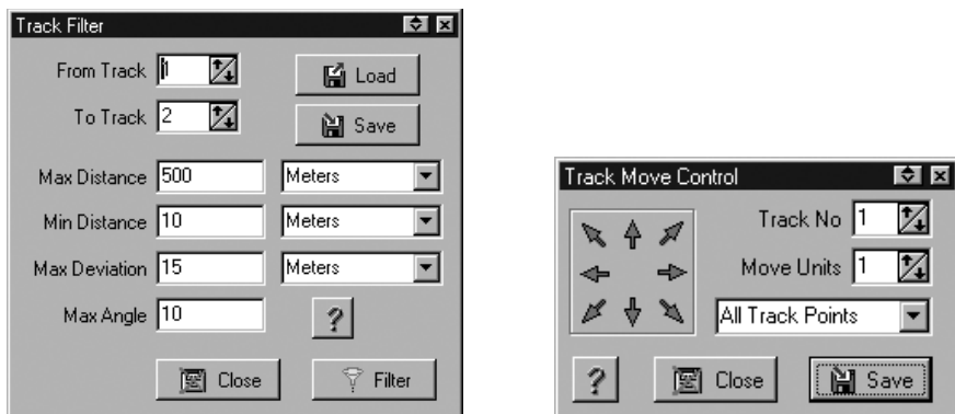
Рис. 3.12. Окна фильтрации (а) и модификации трека (б)
